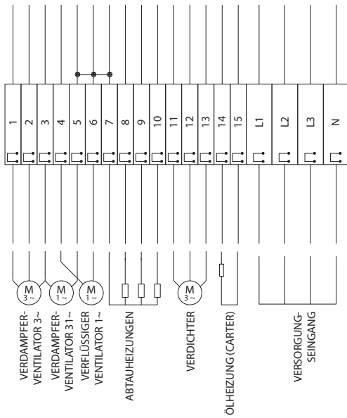
Klemmleiste XP1
